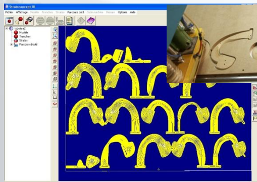
Génération automatique des parcours outil
