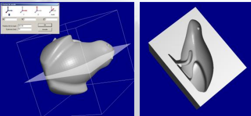
Figure 7 : Création de moule à partir du modèle
