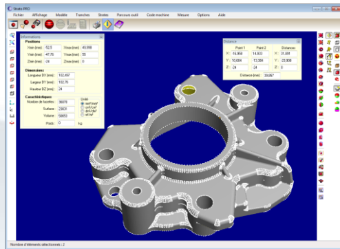
Figure 9 : Caractéristiques du modèle
