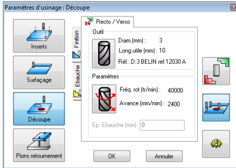
Figure 20 : Outils choisis dans la base de données
