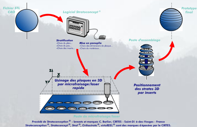
Figure 24 : Schéma de principe du procédé
