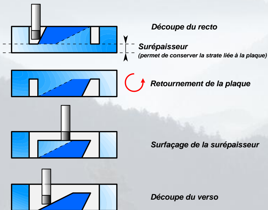
Figure 19 : Retournement et usinage Recto/Verso
