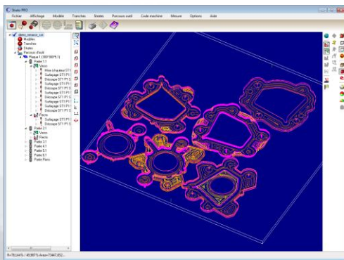
Figure 21 : Parcours d'outil
